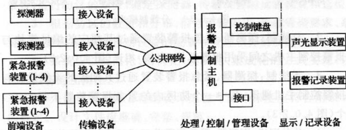
图 4.0.2-4 公共网络模式
