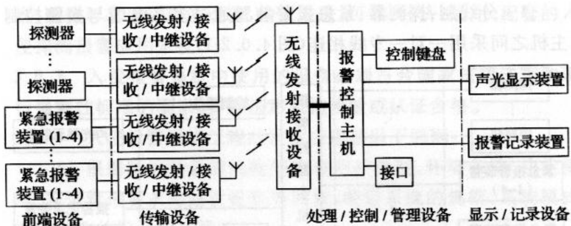
图 4.0.2-3 无线制模式
