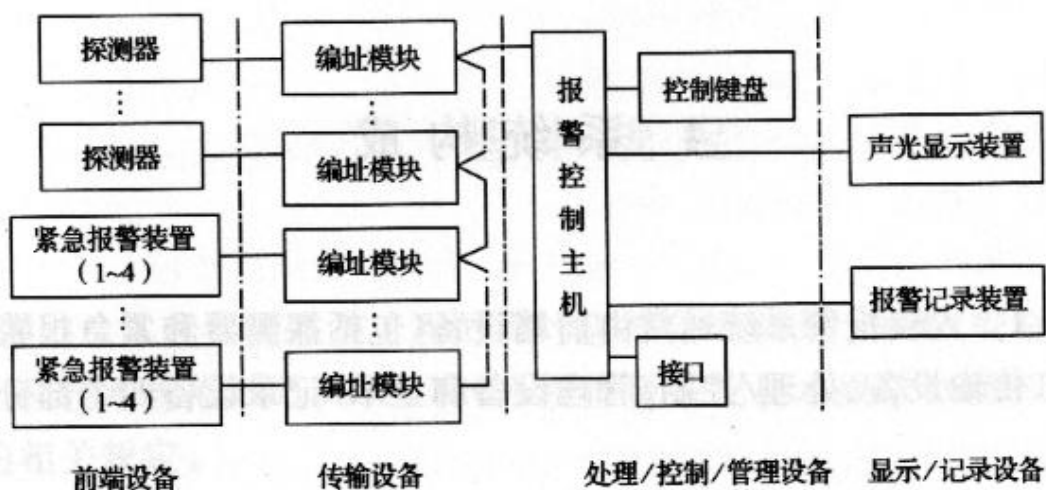
图 4.0.2-2 总线制模式
