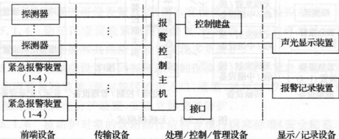
图 4.0.2-1 分线制模式
